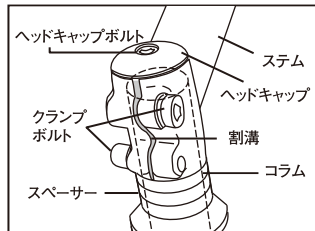
ヘッドセット
